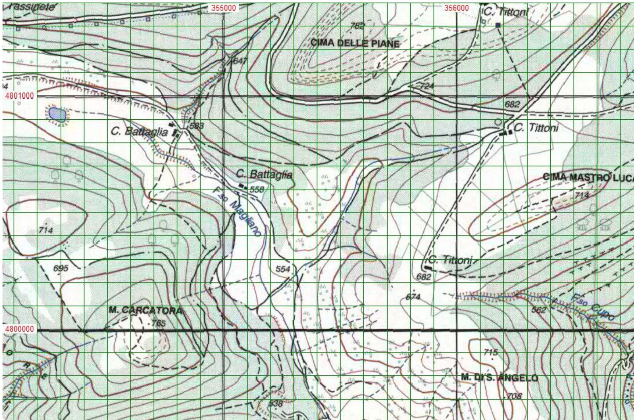
"IL BRANCO" SOFTAIR ANCONA - CAMPO CINGOLI - SCALA 1:10.000 - UTM ED1950 - ISOIPSE 25 M
